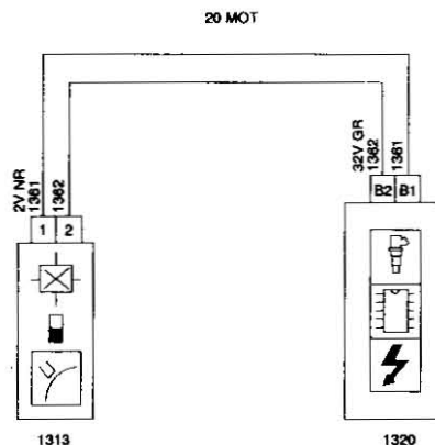
1313 CAPTADOR RÉGIMEN MOTOR (MOTOR TU5JP4 VERSIÓN EUROPA)
