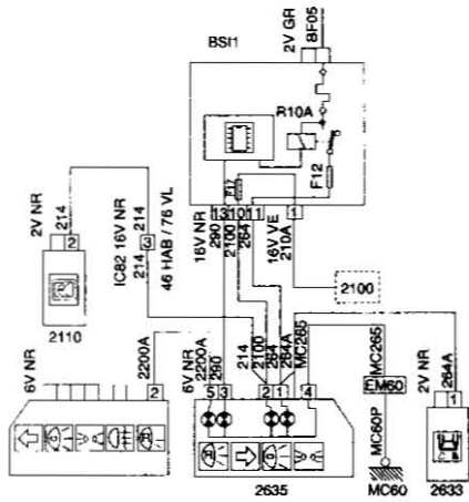
2635 PILOTO TRASERO DERECHO EN CARROCERÍA
