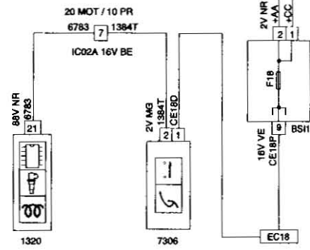
7306 CONTACTOR DE SEGURIDAD DEL REGULADOR DE VELOCIDAD (EMBRAGUE) (MOTOR DW10TD CALCULADOR BOSCH PARA DW10/DW12)
