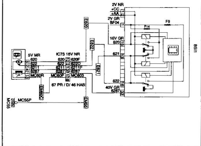
6220 CONTACTOR DE CONDENACIÓN PUERTAS
