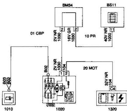
1020 ALTERNADOR (MOTOR TU5JP VERSIÓN EUROPA)
