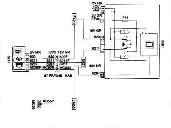
6217 CONJUNTO CERRADURA PUERTA TRASERA DERECHA (SUPERCONDENACIÓN)
