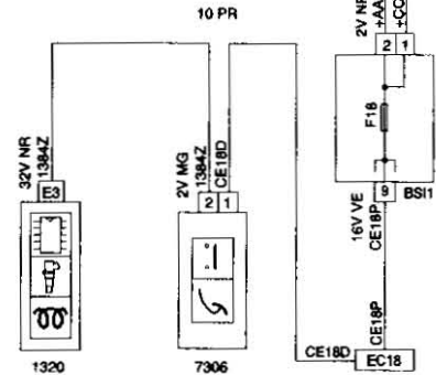
7306 CONTACTOR DE SEGURIDAD DEL REGULADOR DE VELOCIDAD (EMBRAGUE) (MOTOR DW10TD CALCULADOR SIEMENS PARA DW10)
