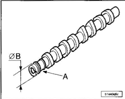
A.- Asiento de junta de árbol de levas.
