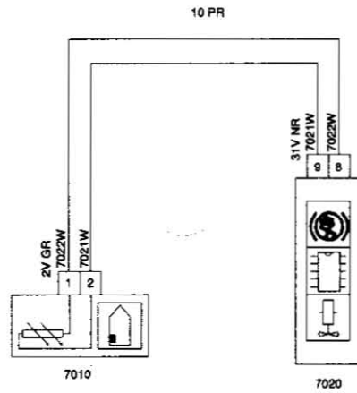
7010 CAPTADOR ANTIBLOQUEO DE RUEDA TRASERA IZQUIERDA
