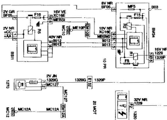
1270 RESISTENCIA RECALENTAMIENTO CARBURADOR O CAJETÍN MARIPOSA (MOTOR EW10J4 - ANTICONTAMINACIÓN L4)
