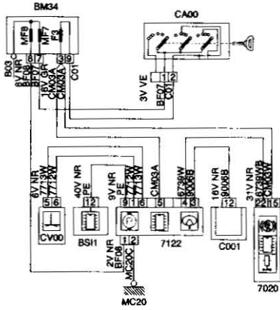
7122 GRUPO ELECTROBOMBA DIRECCIÓN ASISTIDA
