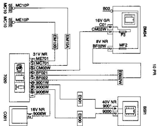
7020 CALCULADOR ANTIBLOQUEO DE RUEDA
